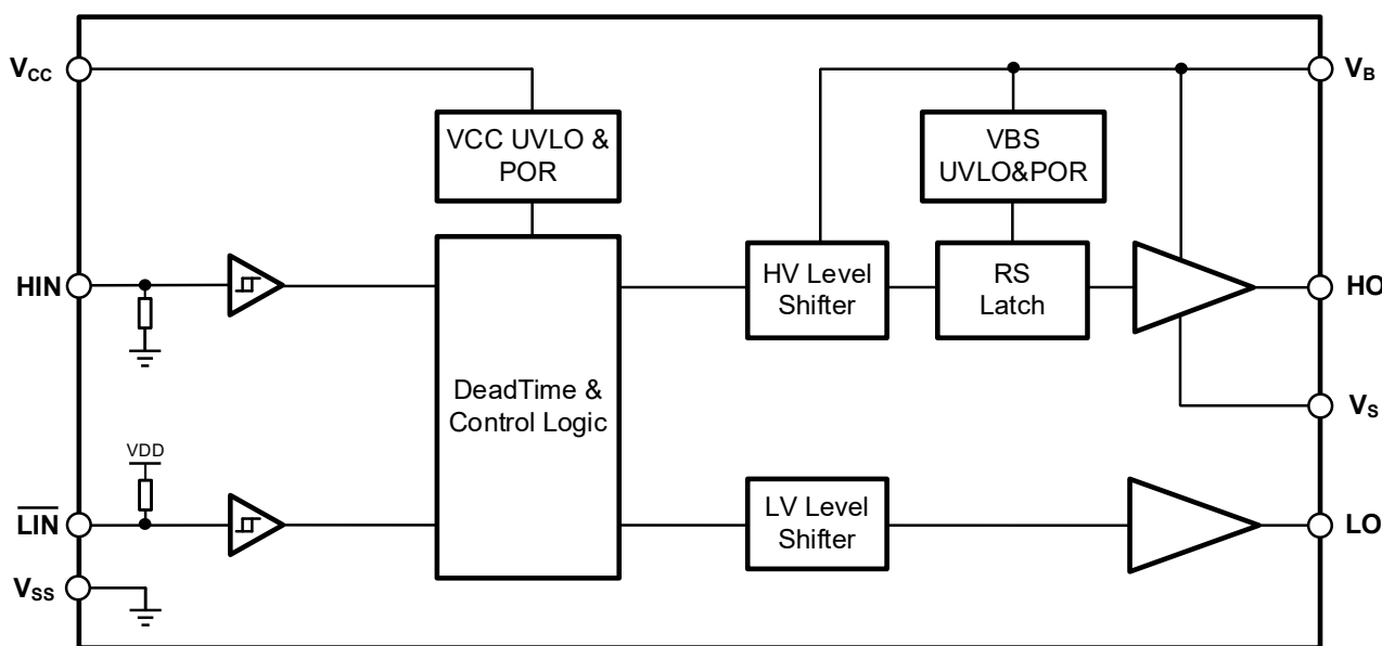
图 10-1 HM2103K 功能框图
