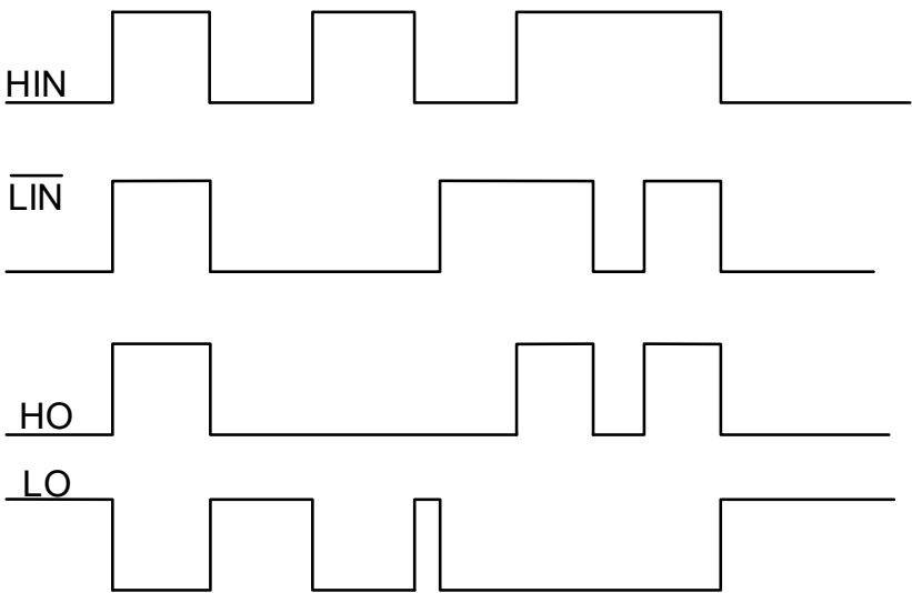
图 9-1 HM2103K 输入输出时序波形
